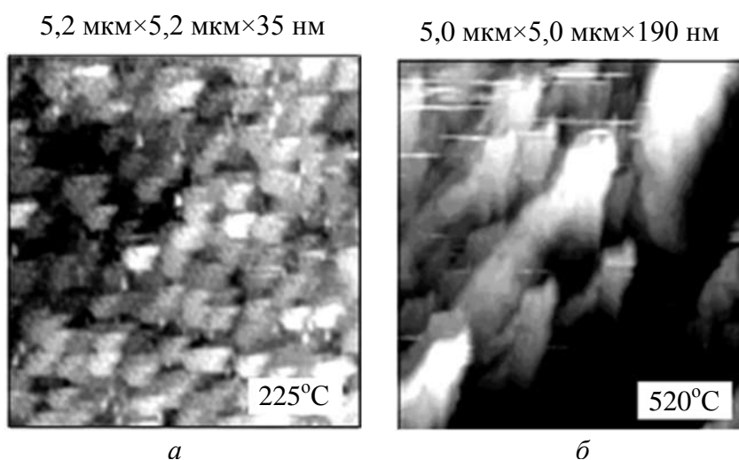
Рис. 6. Изменение структуры углеродных нанокластерных пленок в зависимости от температуры подложки
