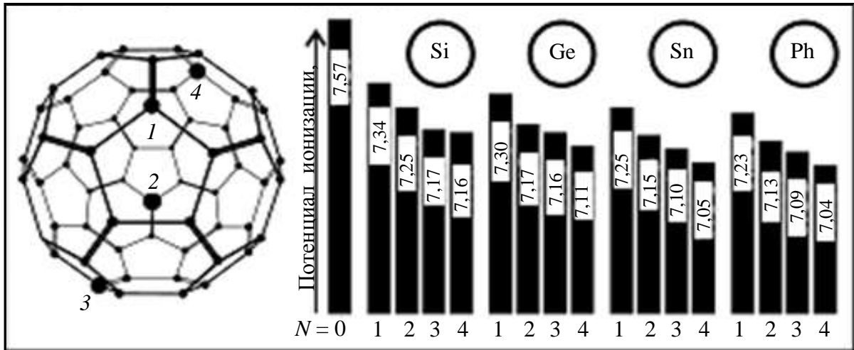
Рис. 3. Фуллерен C_{60-N}X_N
