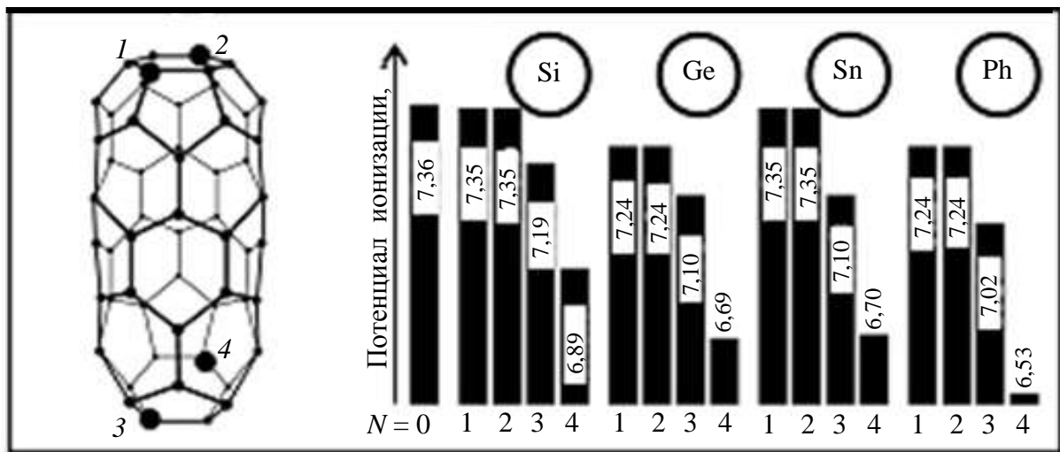
Рис. 4. Нанотрубка C_{60-N}X_N
