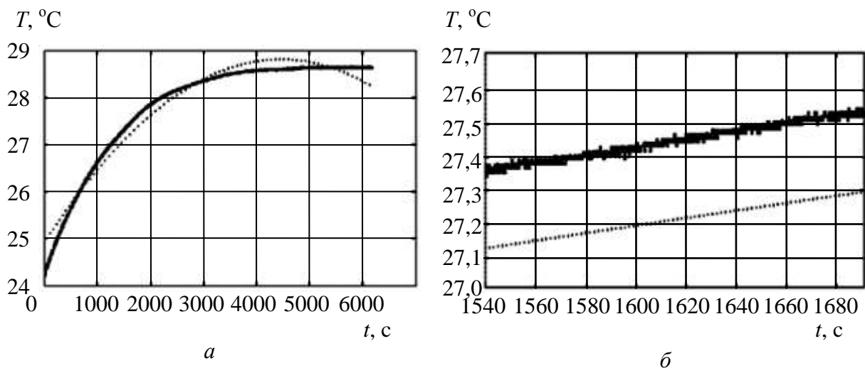
Рис. 4. Зависимость T(t) , полученная с помощью АДТ (полином 2-го порядка): a – в заданном диапазоне изменения параметров; b – в узком диапазоне изменения параметров
