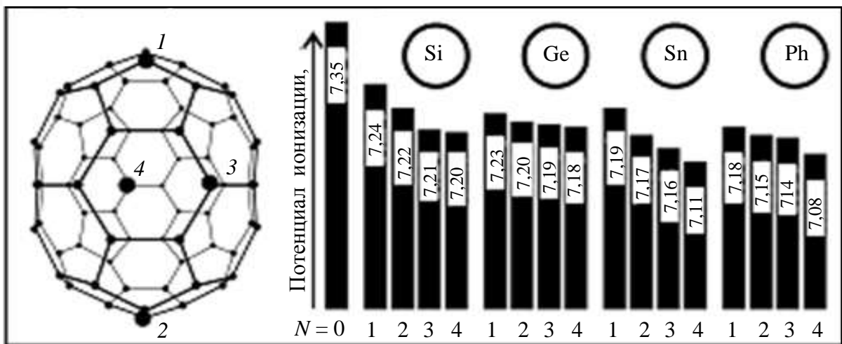
Рис. 5. Фуллерен C_{70-N}X_N
