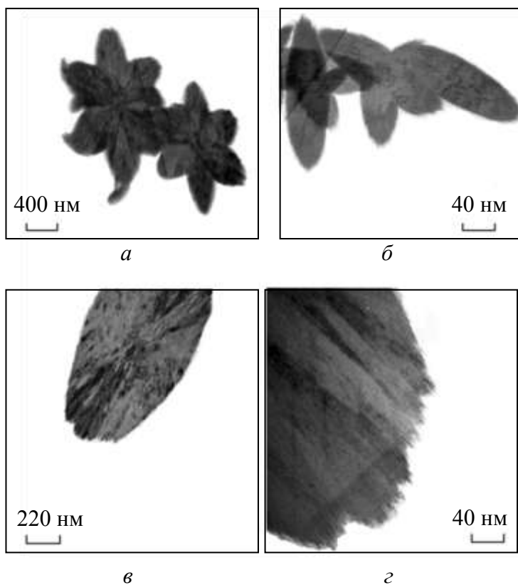
Рис. 1. Изображения, полученные на просвечивающем электронном микроскопе: а – расщепленный сфероидный нанокластер; б и в – плоские кластеры-чешуйки; г – упаковка нанотрубок в нанокластере
